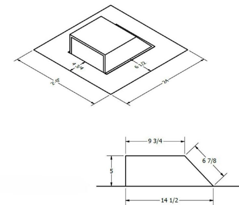
750 VENT
